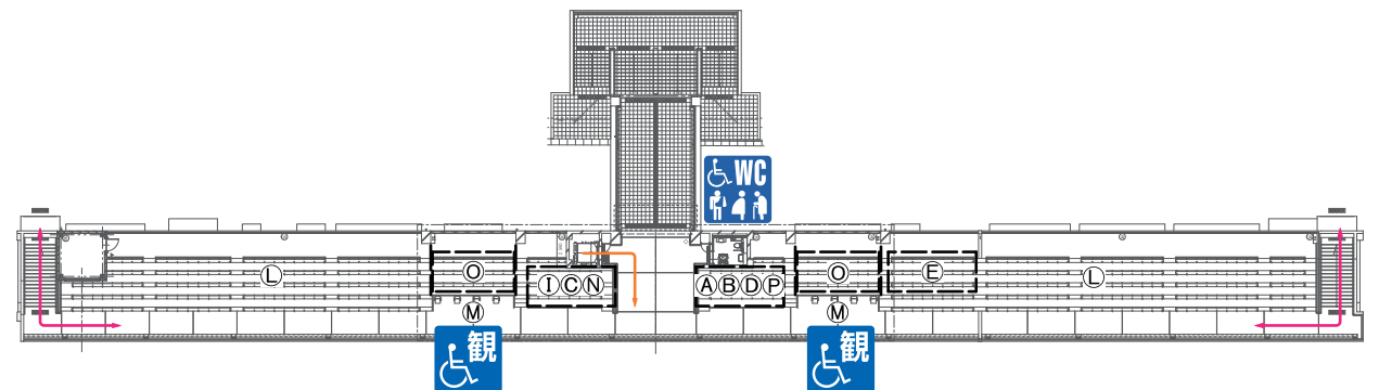
2階平面図
